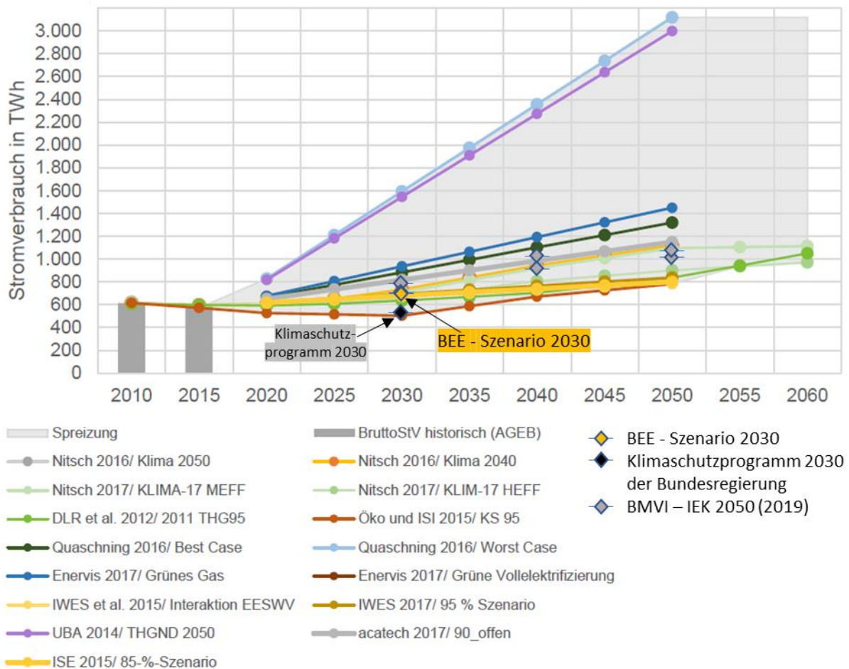
Abb. 4: Projektionen des Bruttostromverbrauchs in aktuellen Energiesystemstudien 18
